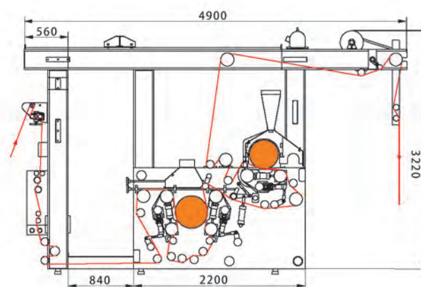
SME472F 双辊三次双面烫光机
