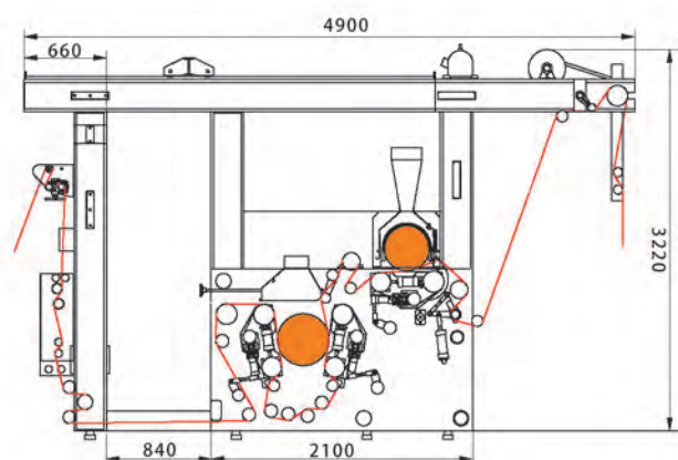
SME472D 双辊三次单面烫光机
