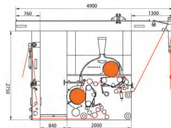
SME472YQ 燃气双辊烫光机 走布图
